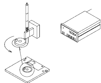
磁碟轉盤偏擺量測
